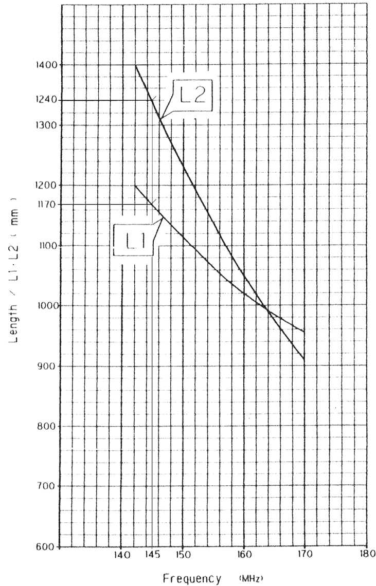
CP-22E CUTTING CHART
